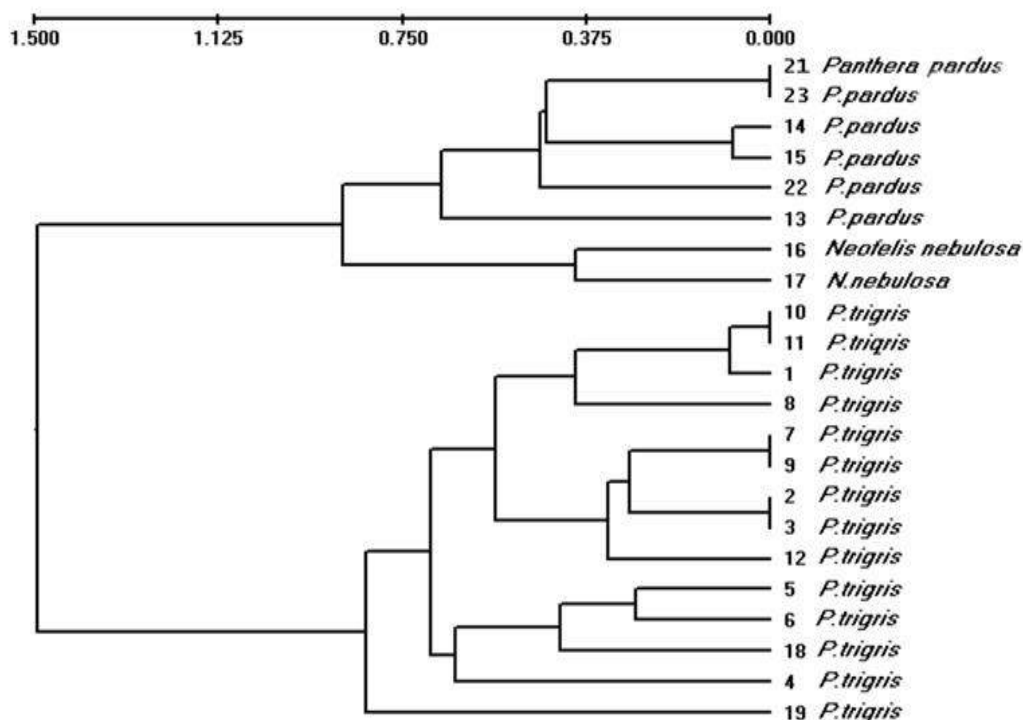
ภาพที่ 25.4 แผนผังความสัมพันธ์ทางพันธุกรรมระหว่างประชากรเสือโคร่ง เสือดาว เสือลายเมฆ จากการจัดกลุ่มโดยวิธี UPGMA ด้วยโปรแกรม TFPGA version 1.3 (ที่มา: สุจิตรา และ พิษณุกร, 2552)
