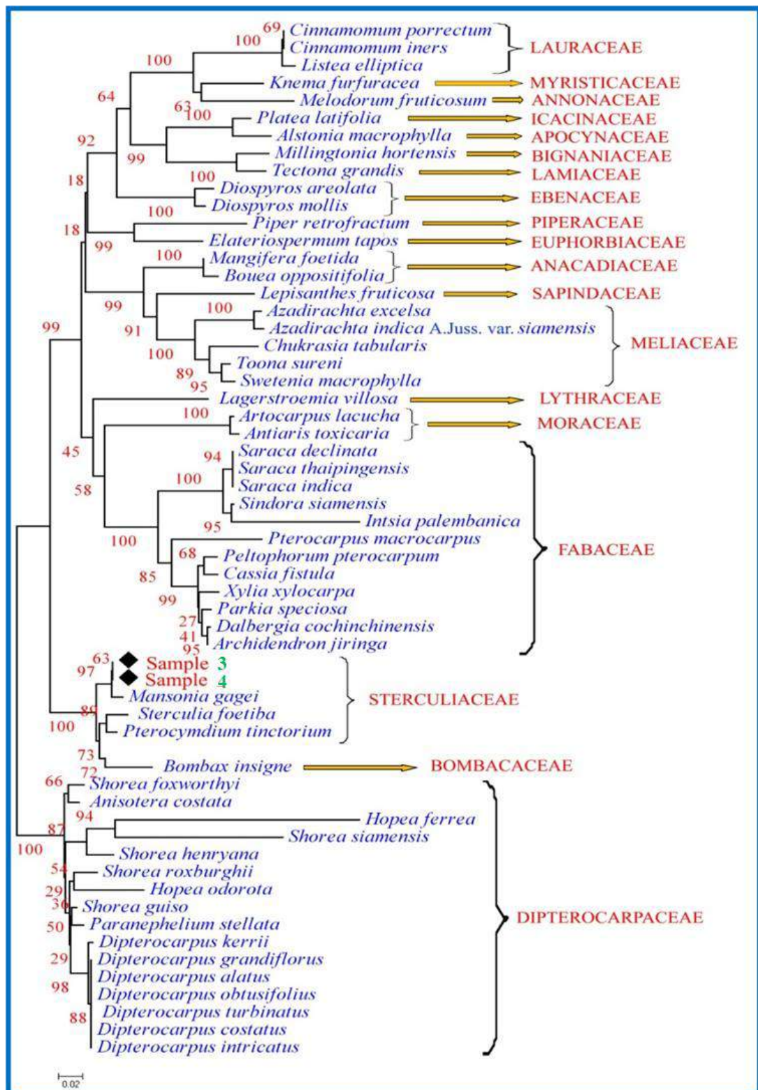
ภาพที่ 18.1 Phylogenetic tree แสดงความสัมพันธ์ทางพันธุกรรมจากตัวอย่างเชื้อที่เลี้ยงกับพรรณไม้ที่มีในฐานข้อมูล (genbank) ในยีน Maturase k (Mat K) (ที่มา: สุจิตรา, 2560)
