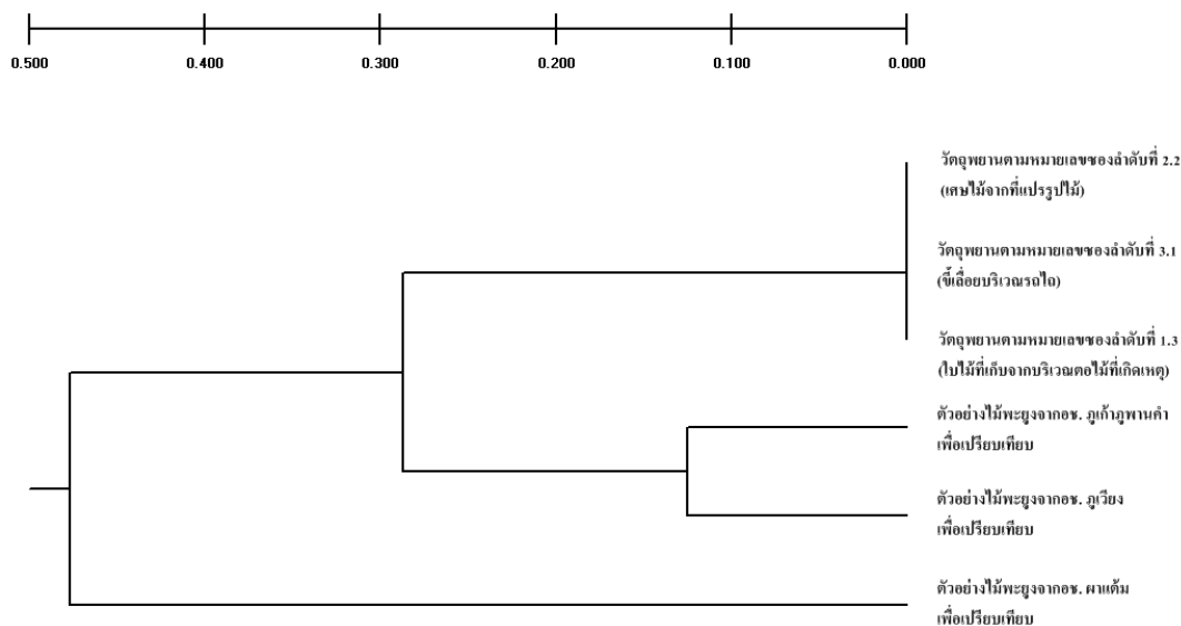
ภาพที่ 24.3 แผนภาพแสดงความสัมพันธ์ทางพันธุกรรมจากการวิเคราะห์ไมโครแซทเทลไลท์ 10 ตำแหน่งของวัตถุพยานตามหมายเลขของลำดับที่ 1.3 วัตถุพยานตามหมายเลขของลำดับที่ 2.2 วัตถุพยานตามหมายเลขของลำดับที่ 3.1 และตัวอย่างไม้พะยูน ( Dalbergia cochinchinensis ) จากแหล่งอื่นที่ใช้เปรียบเทียบ ที่แสดงให้เห็นว่า วัตถุพยานตามหมายเลขของลำดับที่ 1.3, 2.2 และ 3.1 มีลักษณะทางพันธุกรรมเหมือนกัน
