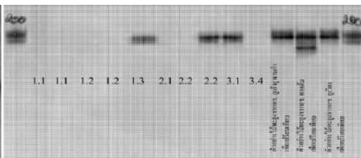
ลายพิมพ์ดีเอ็นเอที่ตำแหน่ง DELB_120
