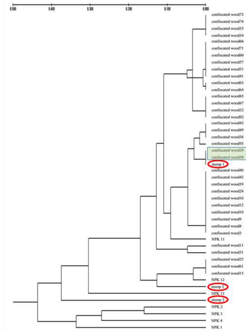
ภาพที่ 22.2 การวิเคราะห์ความสัมพันธ์ทางพันธุกรรมมีเครื่องหมายดีเอ็นเอชนิดไมโครแซทเทลไลท์ 3 ตำแหน่ง ในชิ้นไม้ของกลางของไม้พะยูน ( Dalbergia cochinchinensis ) เปรียบเทียบกับต่อไม้ 3 ต่อ ที่ถูกลักลอบตัดอย่างผิดกฎหมาย และต้นพะยูน ( D. cochinchinensis ) 7 ต้นจากอุทยานแห่งชาติน้ำพอง จ.ขอนแก่น ได้แสดงให้เห็นว่าไม้ชิ้นที่ 23 และ 30 มีลักษณะพันธุกรรมตรงกับ ต่อไม้ที่ถูกลักลอบตัดต่อที่ 1 (ที่มา: สุจิตรา, 2560)
