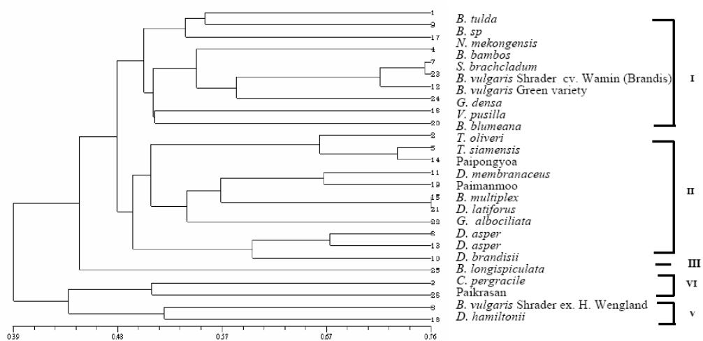
ภาพที่ 8.2 การจัดกลุ่มความสัมพันธ์ทางพันธุกรรมของไผ่ 26 ชนิด ในลักษณะ Phylogenetic tree (ที่มา: รังสัน และ สุจิตรา, 2548)
