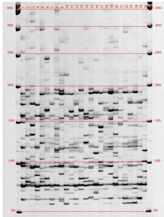
ภาพที่ 8.1 ลายพิมพ์ดีเอ็นเอที่เกิดจากคู่ไพรเมอร์ E-AGG/M-CTC ของไผ่ 26 ชนิด (ที่มา: รังสัน และ สุจิตรา, 2548)
