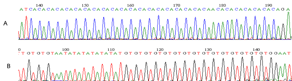
ภาพที่ 3.2 แสดงส่วนที่เป็นไมโครแซทเทลไลต์ซึ่งพบในไม้พะยูน (A) แสดงส่วนที่เป็นชุด CA 27 ซ้ำ (B) แสดงส่วนที่เป็นชุด TA 7 ซ้ำและ GT 16 ซ้ำ (ที่มา: สุจิตรา และคณะ, 2552)
