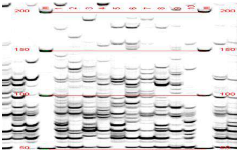
ภาพที่ 9.2 ภาพลายพิมพ์เอเอฟแอลพีของกล้วยไม้รองเท้านารีเหลืองกระบี่ที่ได้จากการทำ electrophoresis โดยใช้เครื่อง Gel-Scan 2000 ในภาพเป็นตัวอย่างลายพิมพ์เอเอฟแอลพี จากการใช้คู่มือพรเมอร์ที่ E-AGC / M-CTC จากแหล่ง อำเภอบะเหลียน จังหวัดตรัง (ที่มา: จักรพันธ์และสุจิตรา, 2548)
