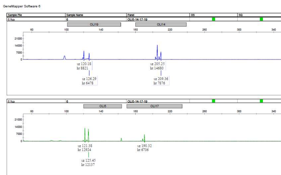
ภาพที่ 12.2 แสดง Electropherogram ที่ผ่านการดีดสียฟลูออเรสเซนและวิเคราะห์ด้วยเครื่อง Genetic Analyzer 3500 ในไม้ชิงชัน ( Dalbergia oliveri ) (ที่มา: สุจิตรา และคณะ, 2564)
