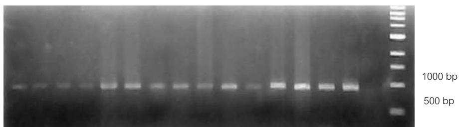
ภาพที่ 16.1 แสดงการตรวจวิเคราะห์ชิ้นดีเอ็นเอขนาด 930 คู่เบส ที่ได้จากการเพิ่มปริมาณด้วยเทคนิคพีซีอาร์โดยใช้ไพรเมอร์จากยีน matK (ที่มา: สัจจิรา, 2554)
